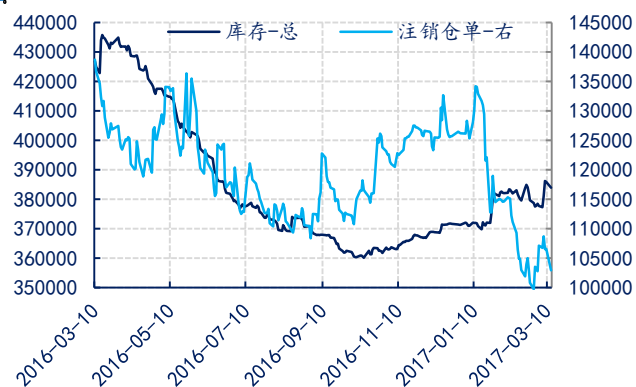
图 52: LME 镍库存与注销仓单
