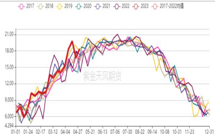
水位-云南溪洛渡水库
