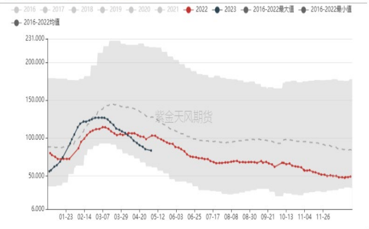
【AL】中国电解铝社会库存-季节性(万吨)
