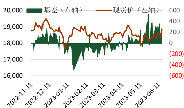
图 11: 基差 (元/吨)
